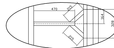
SEÇÃO BB
