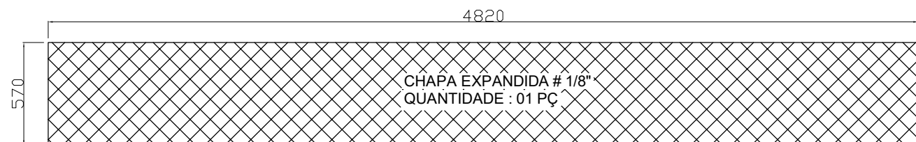
VISTA INFERIOR
