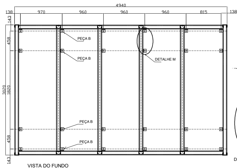
VISTA DO FUNDO
