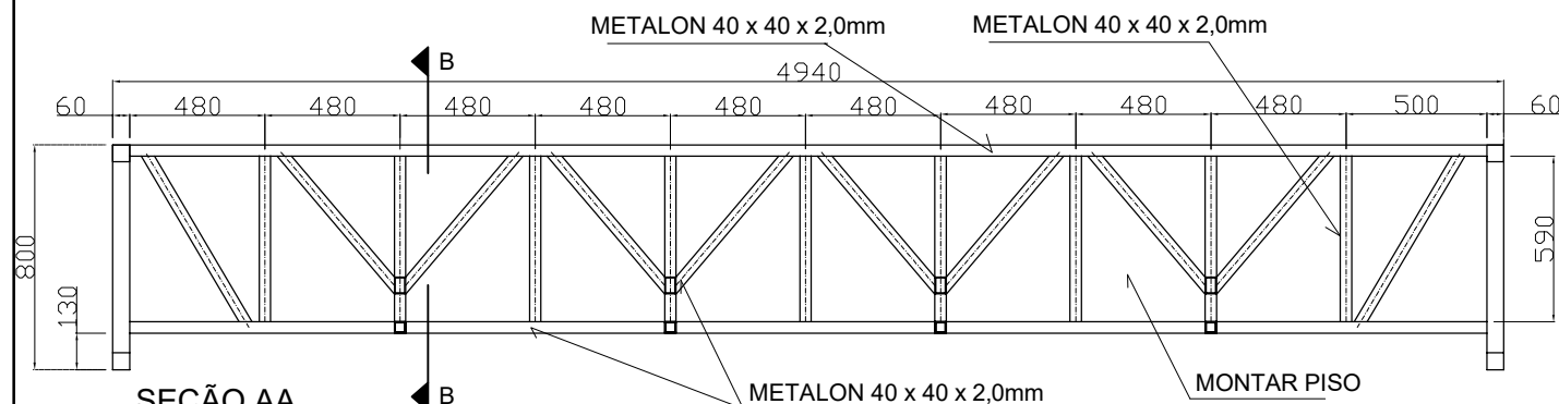
SEÇÃO AA
