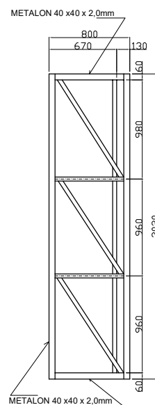
VISTA LATERAL
