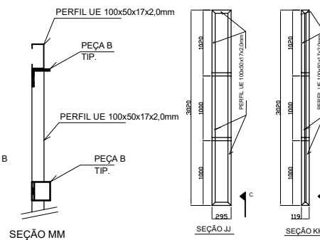
SEÇÃO MM
