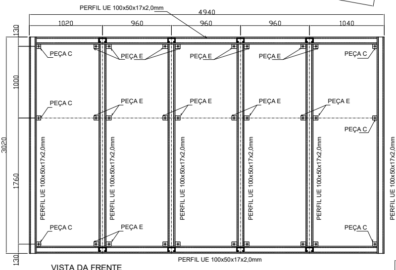
VISTA DA FRENTE
