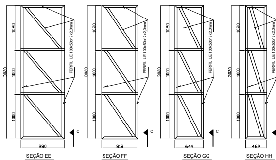
SEÇÃO EE
