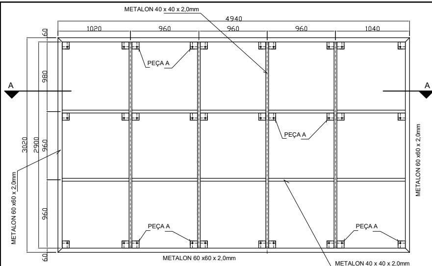
VISTA DO FUNDO
