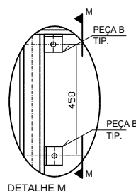
DETALHE M
